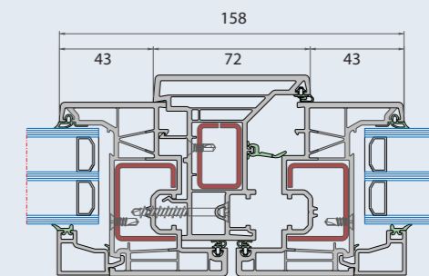
Secção horizontal
