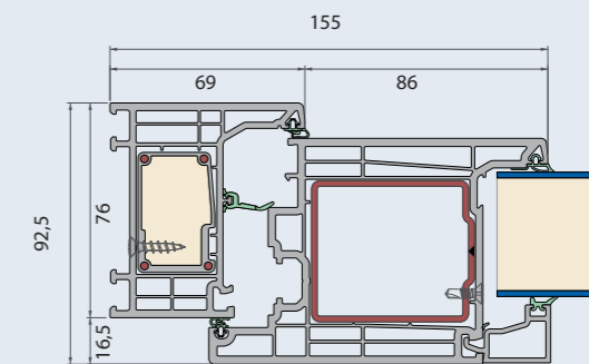
Sección horizontal
